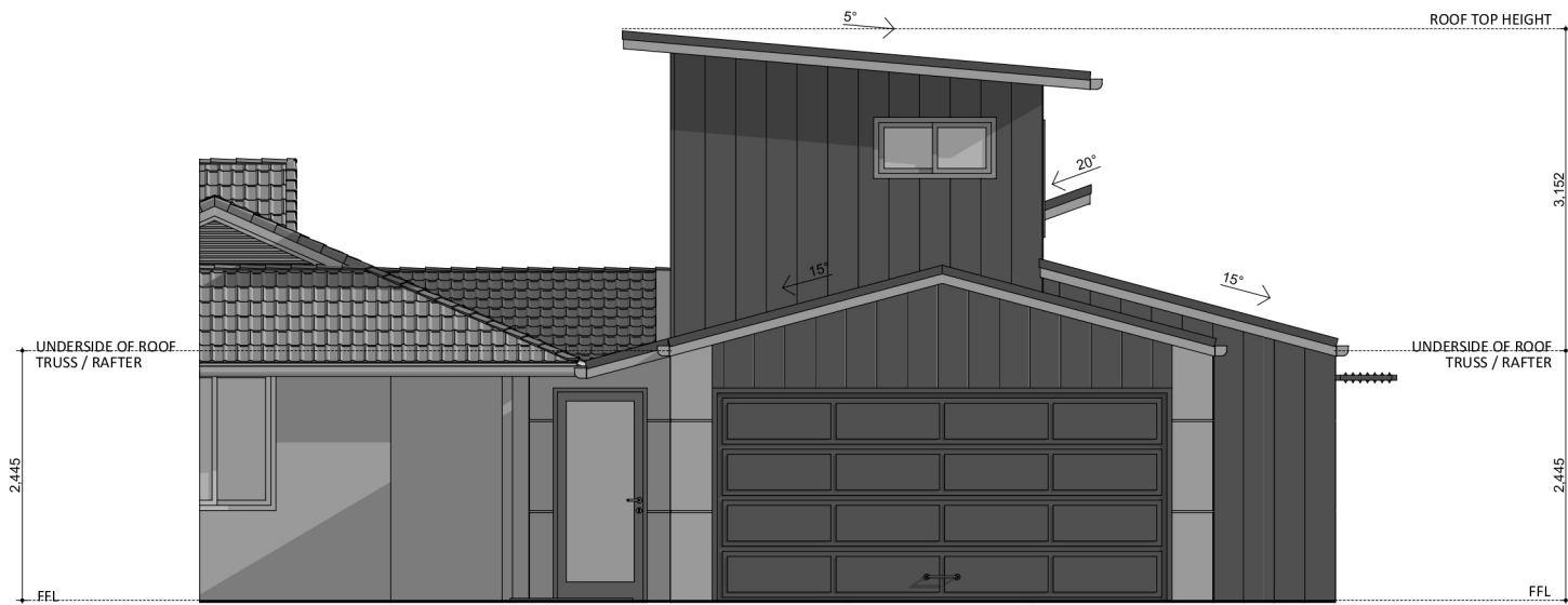
ELEVATION 01
