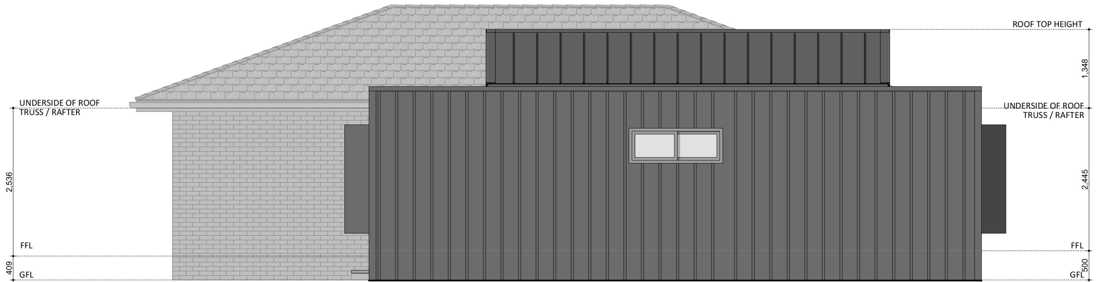
ELEVATION 02
