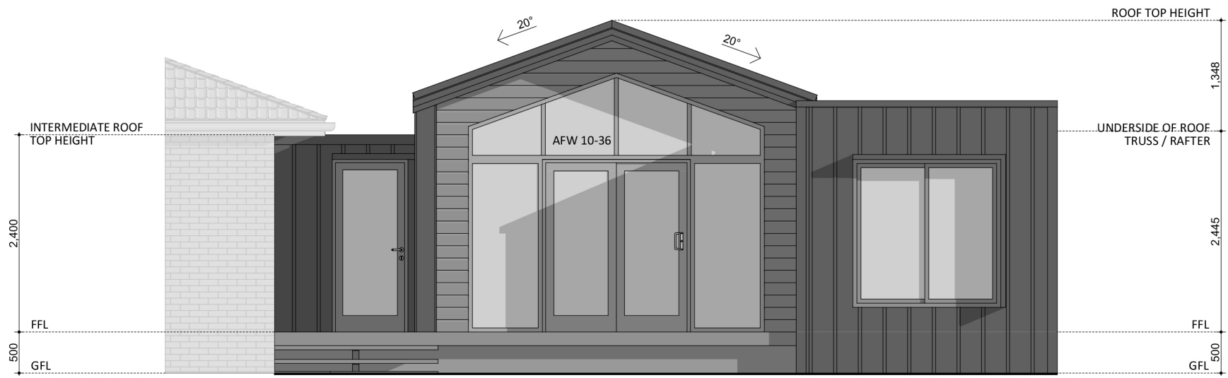
ELEVATION 01
