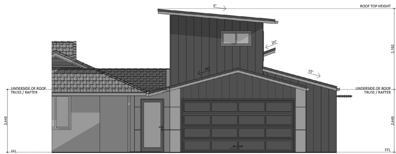
ELEVATION 01
