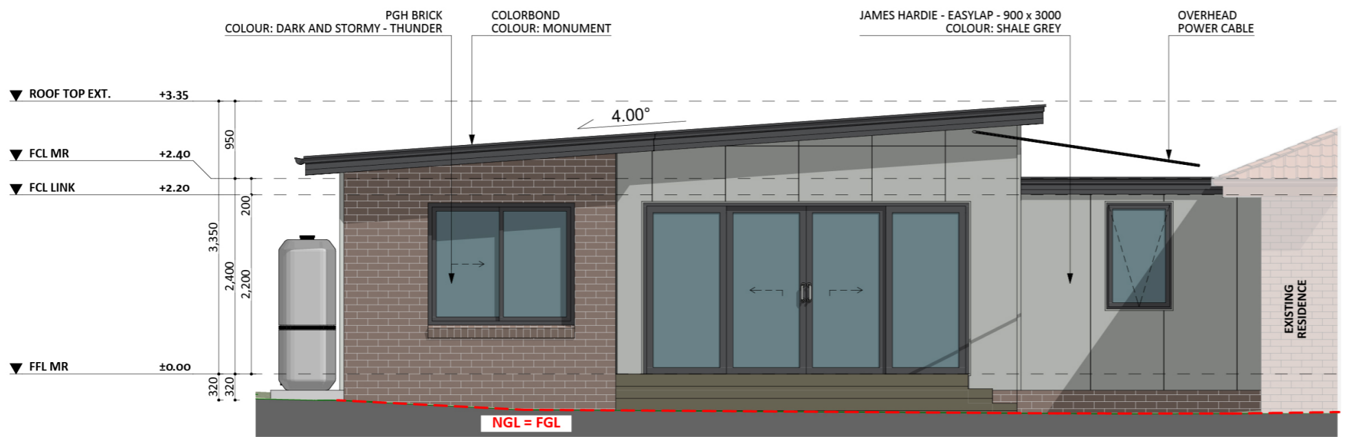
ELEVATION 01
