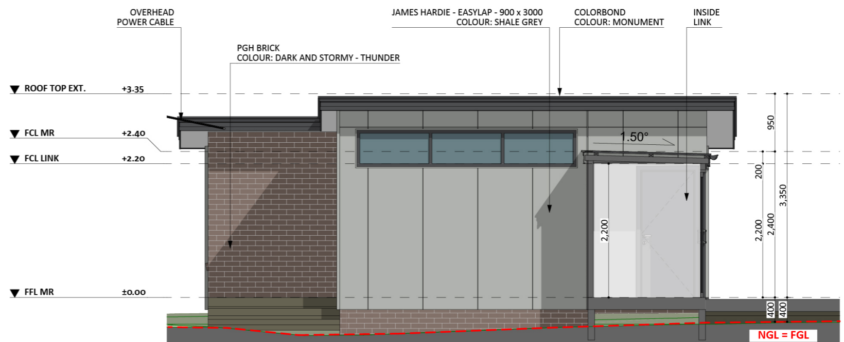
ELEVATION 02
