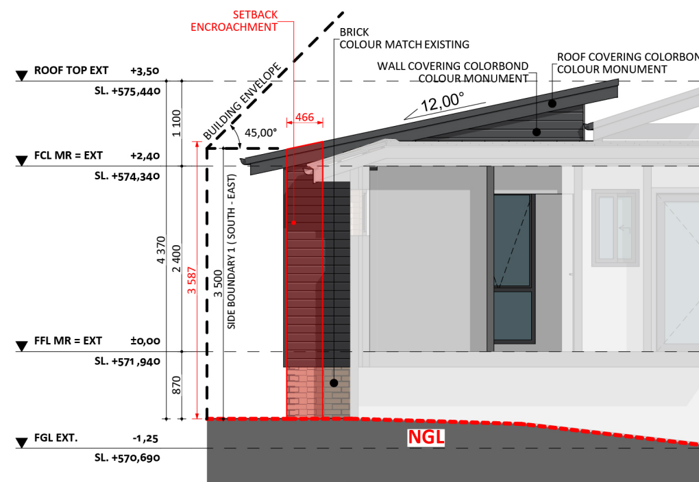
ELEVATION 02
