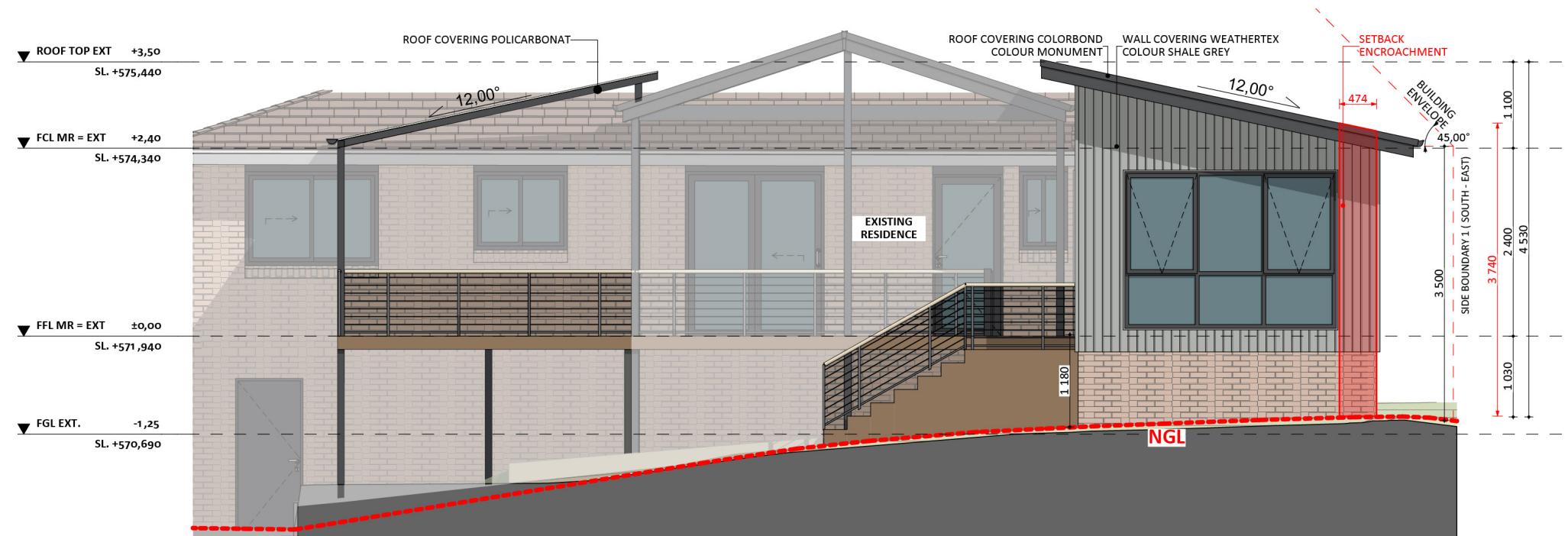
ELEVATION 01
