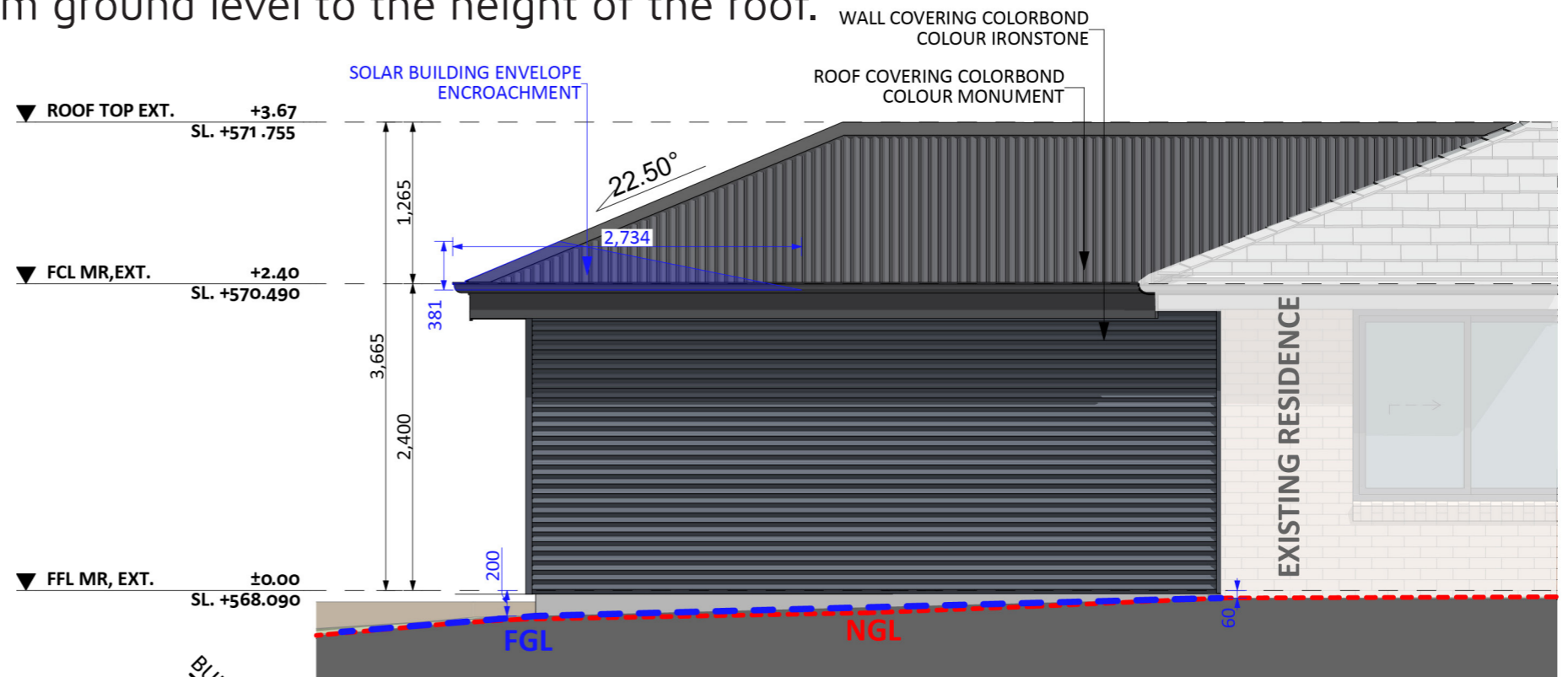
ELEVATION 02
