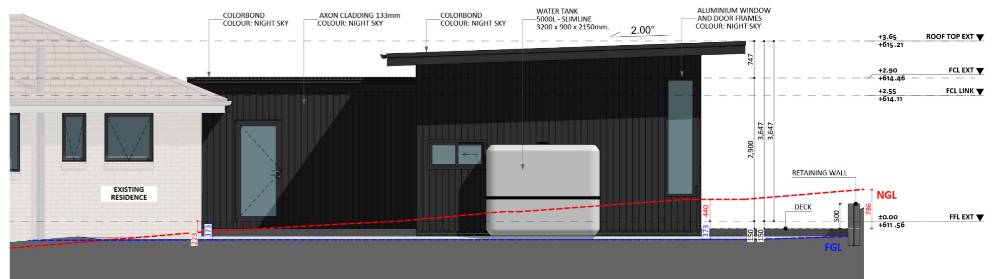
ELEVATION 04
