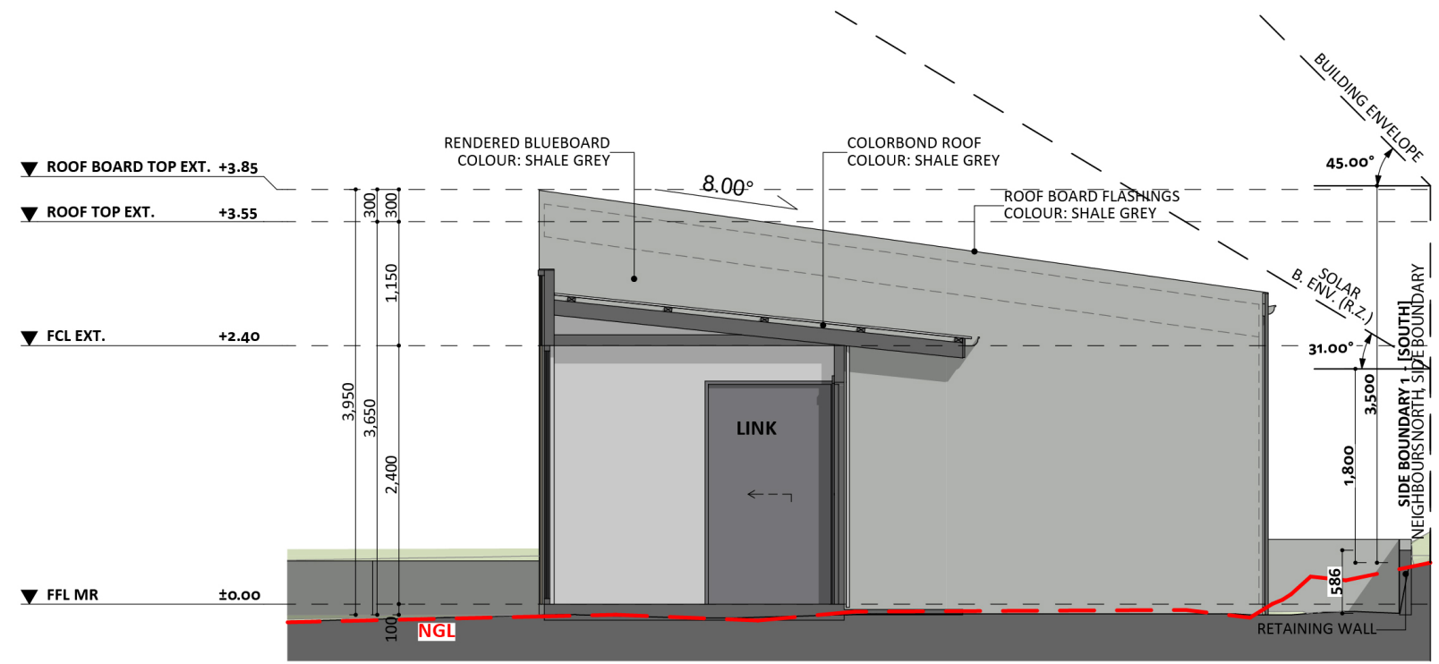
ELEVATION 2
