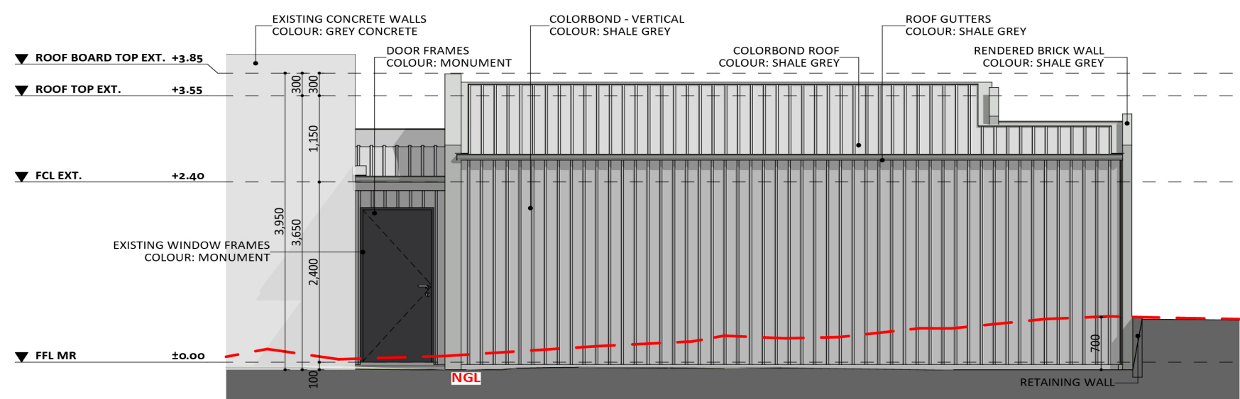
ELEVATION 3
