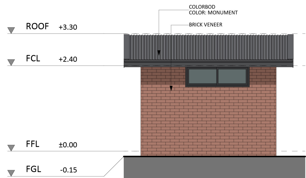
ELEVATION 2
