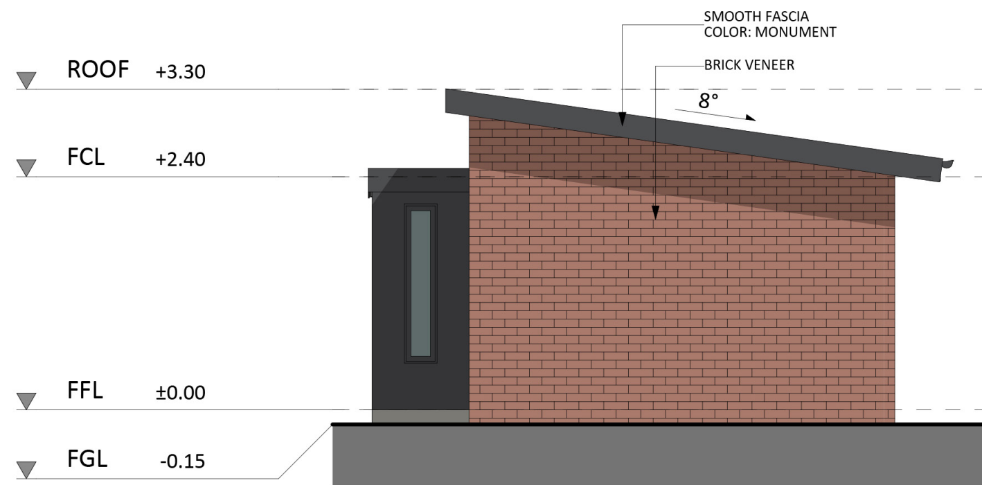
ELEVATION 1
