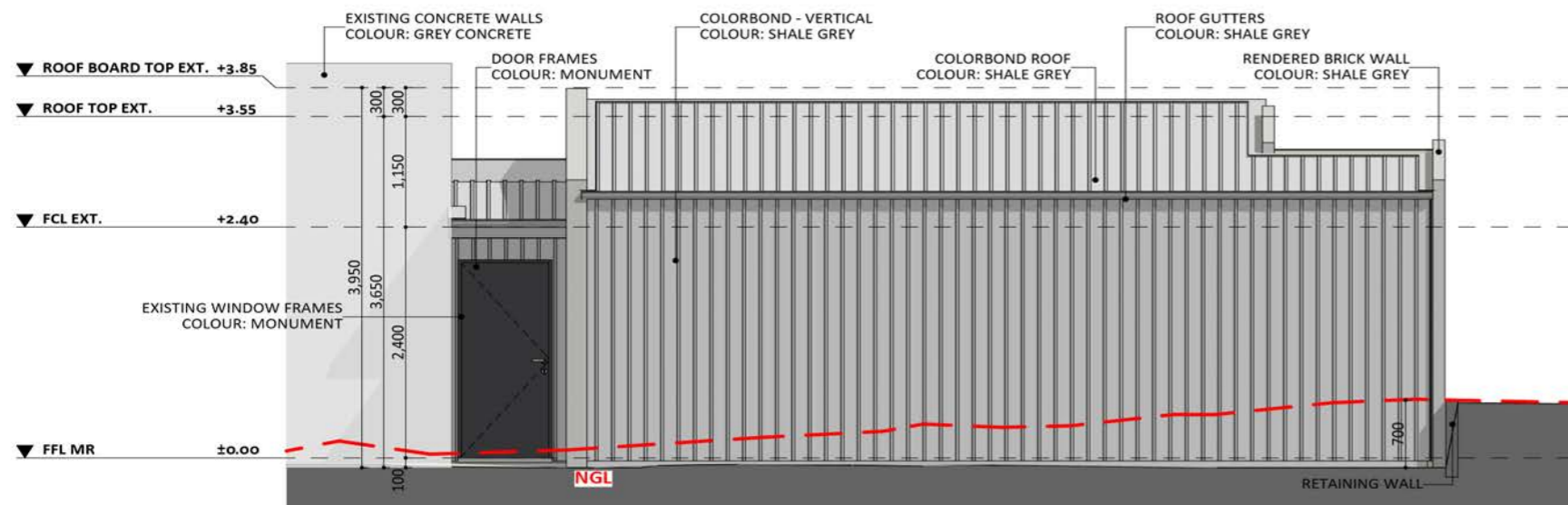
ELEVATION 3
