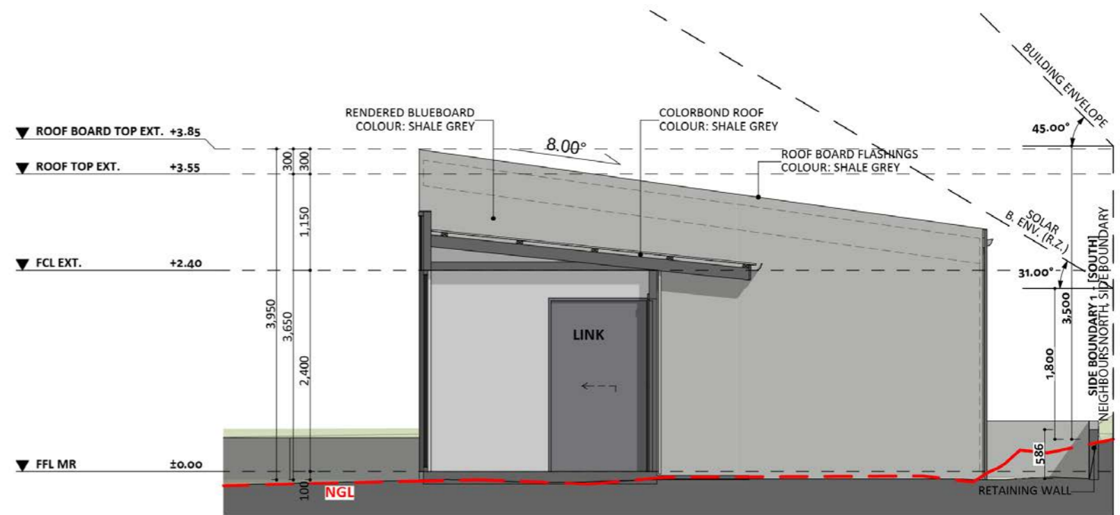
ELEVATION 2
