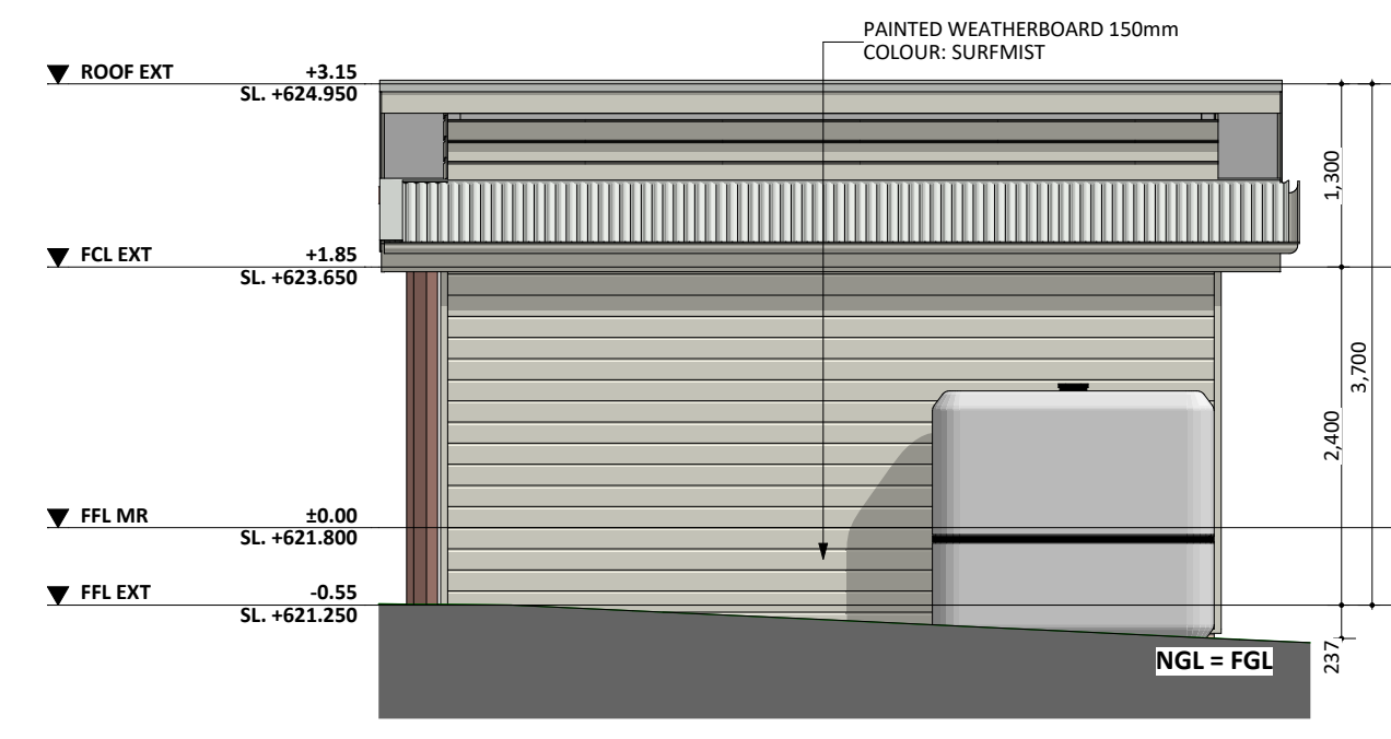
E4 EAST ELEV.
