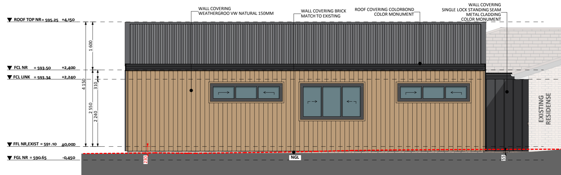
ELEVATION 4
