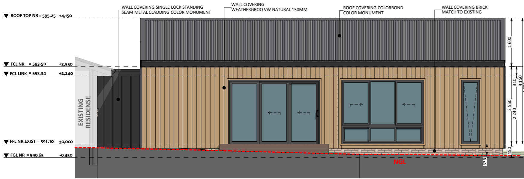
ELEVATION 1
