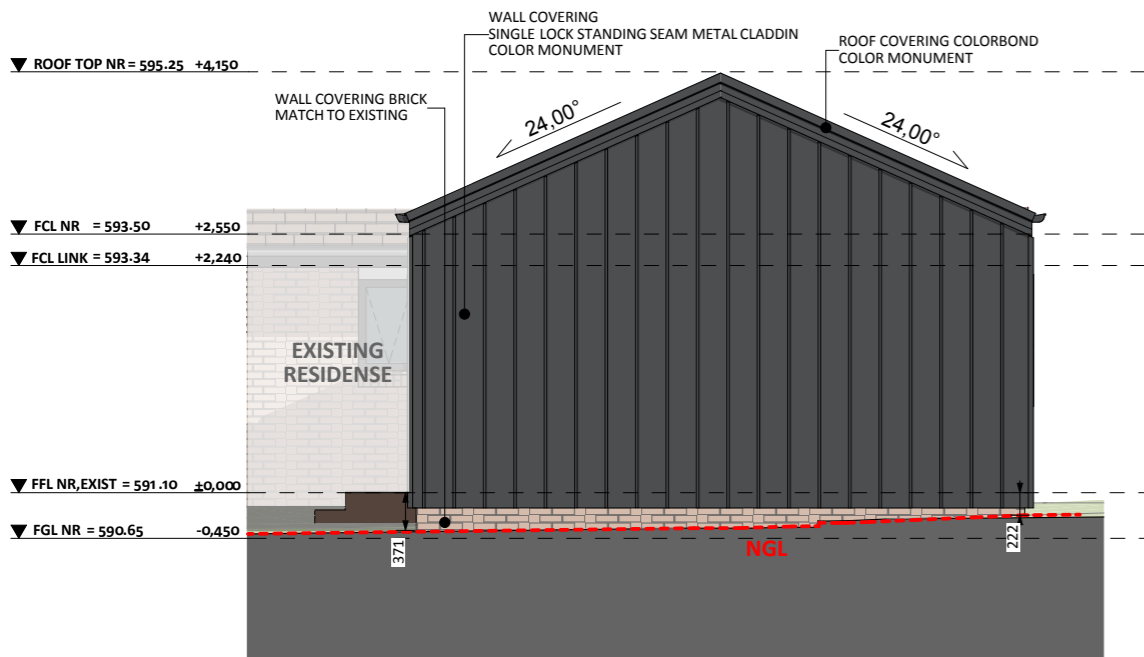
ELEVATION 3
