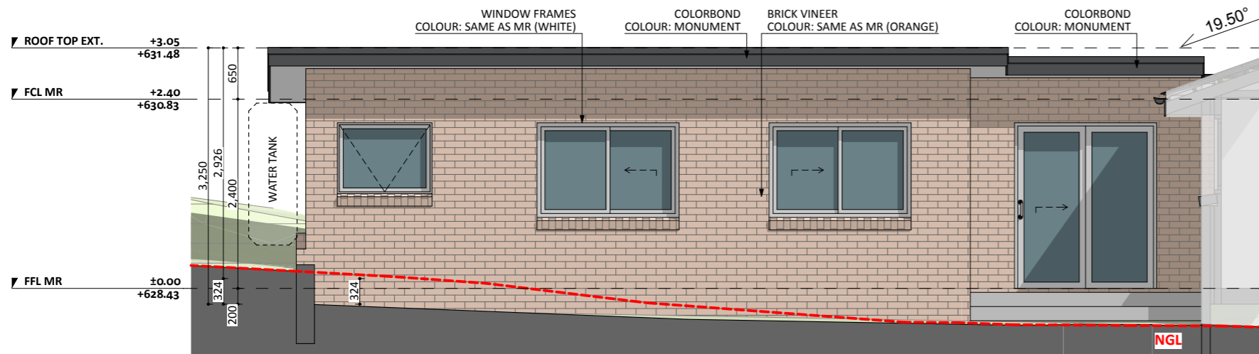
ELEVATION 01
