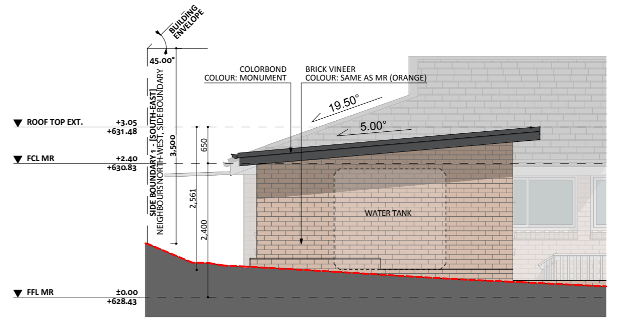
ELEVATION 02
