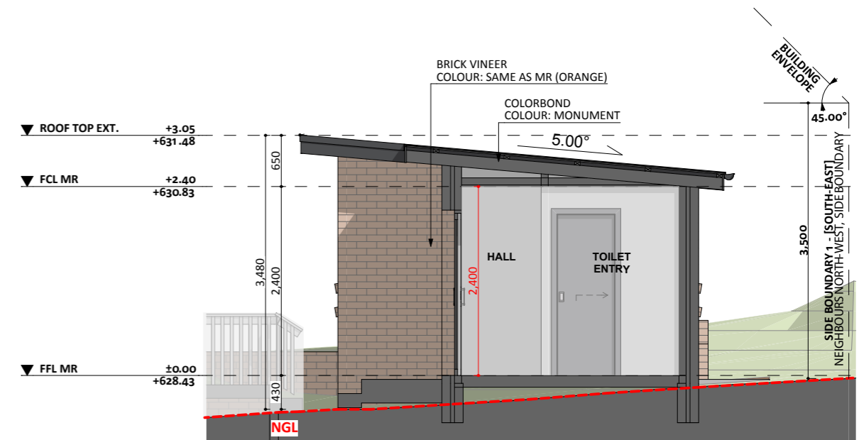
ELEVATION 04
