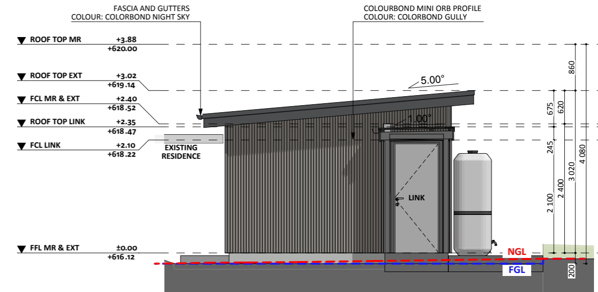
ELEVATION 02
