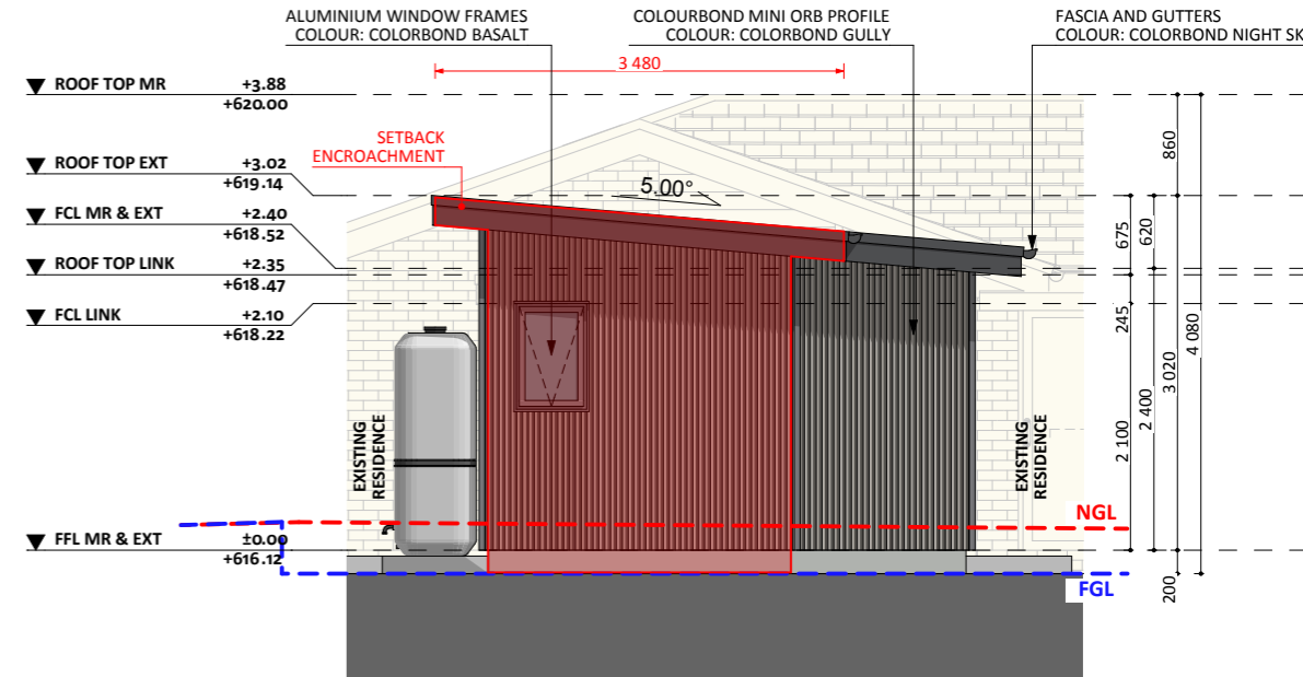
ELEVATION 04
