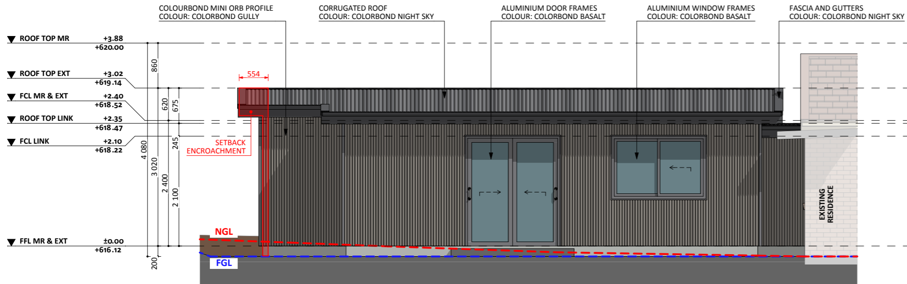
ELEVATION 01
