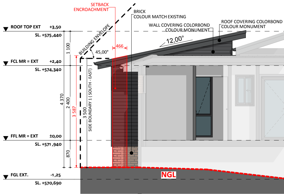
ELEVATION 02
