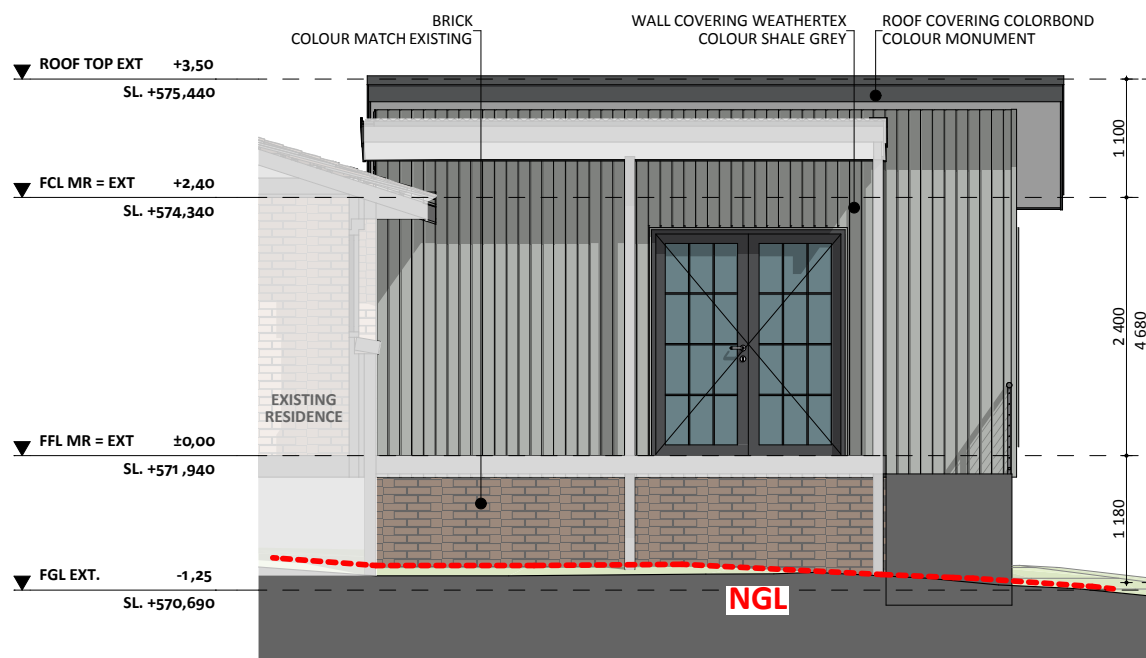
ELEVATION 04
