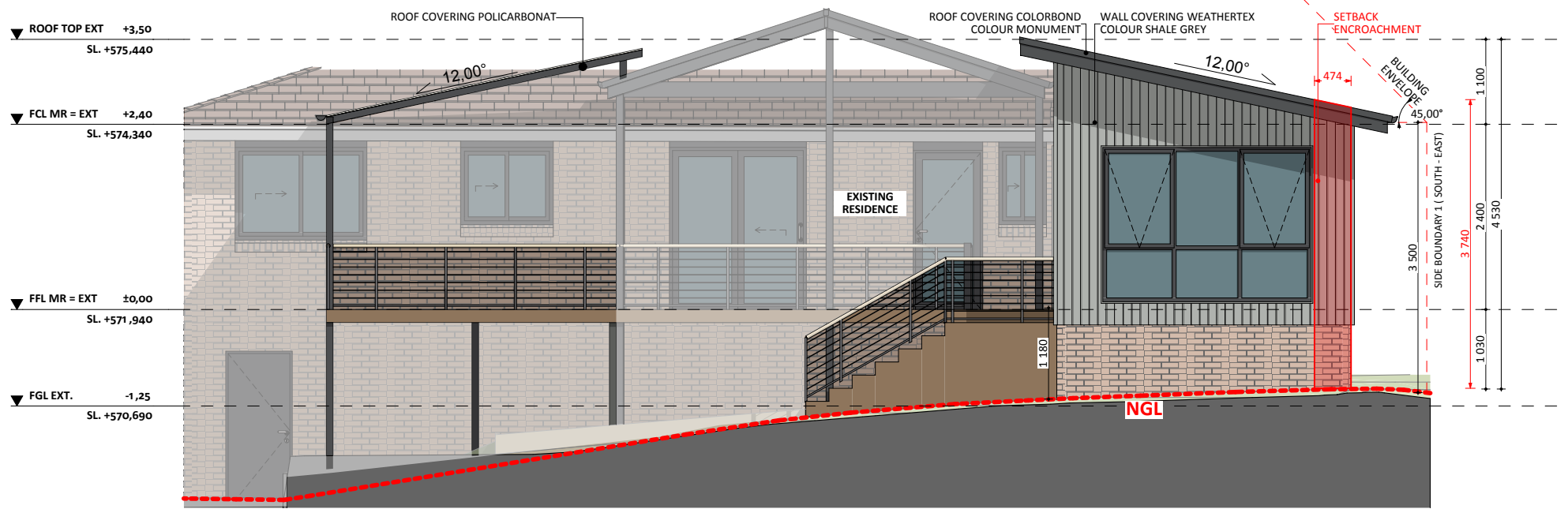
ELEVATION 01
