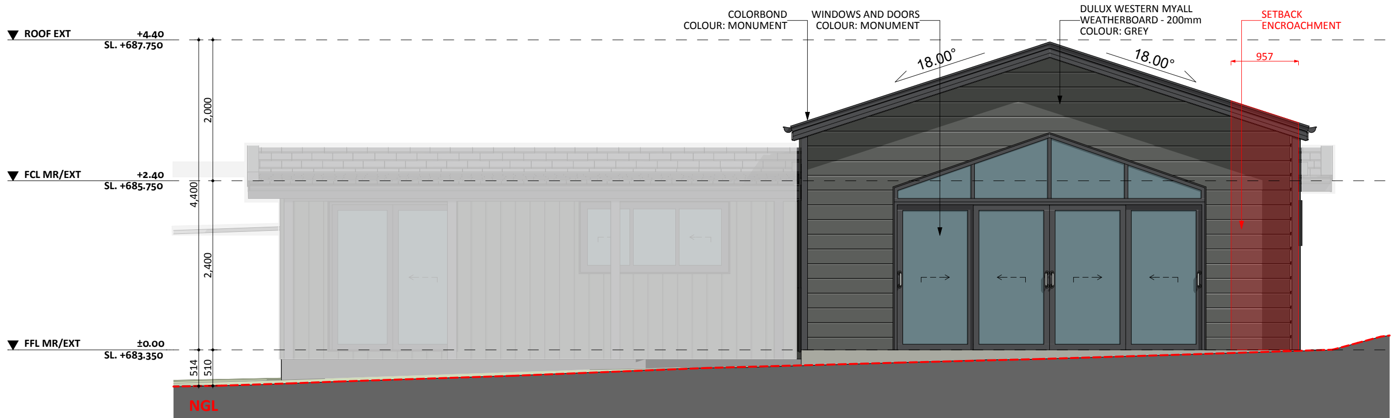
ELEVATION 01
