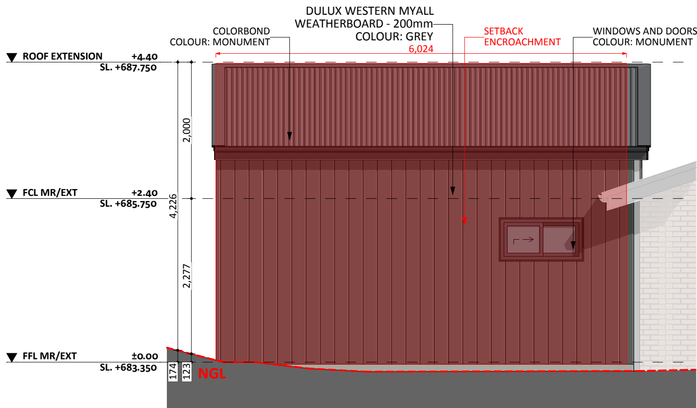
ELEVATION 02
