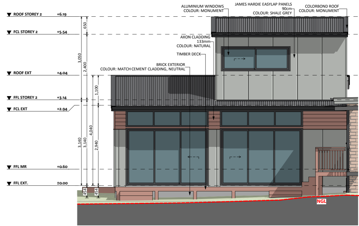
ELEVATION 02
