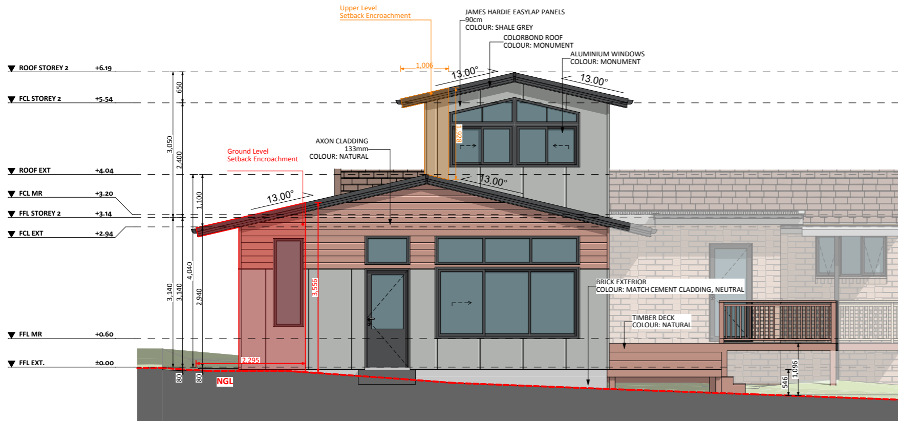
ELEVATION 01
