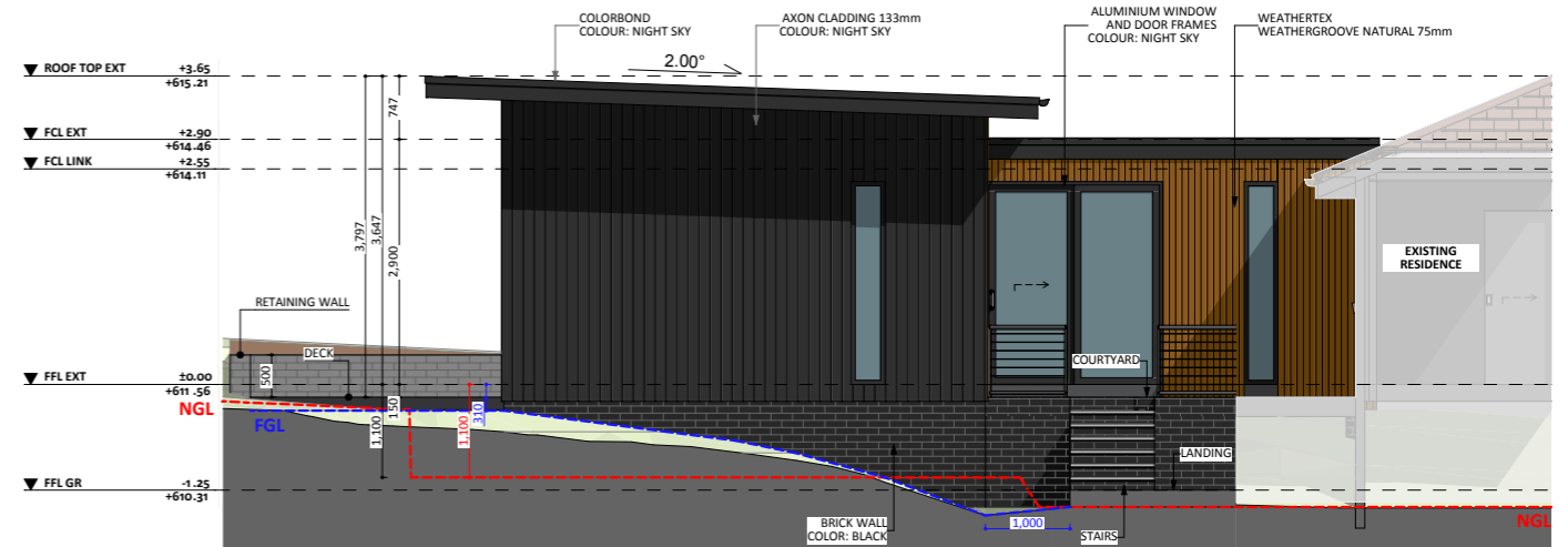
ELEVATION 02
