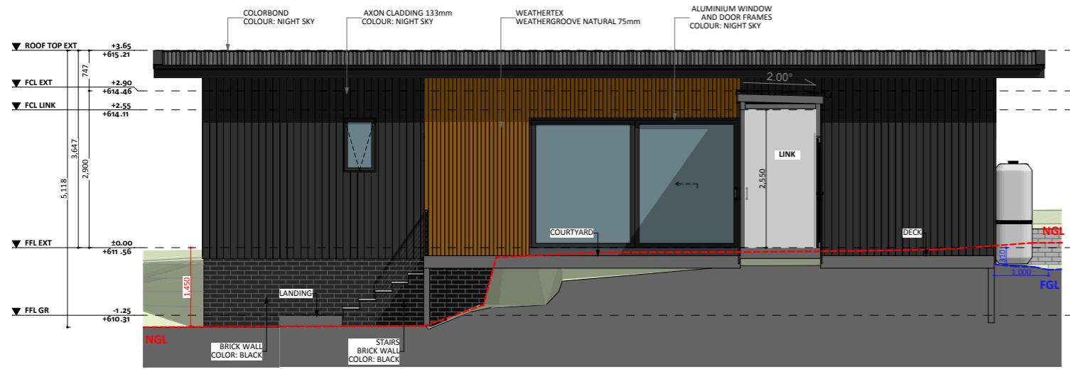
ELEVATION 01
