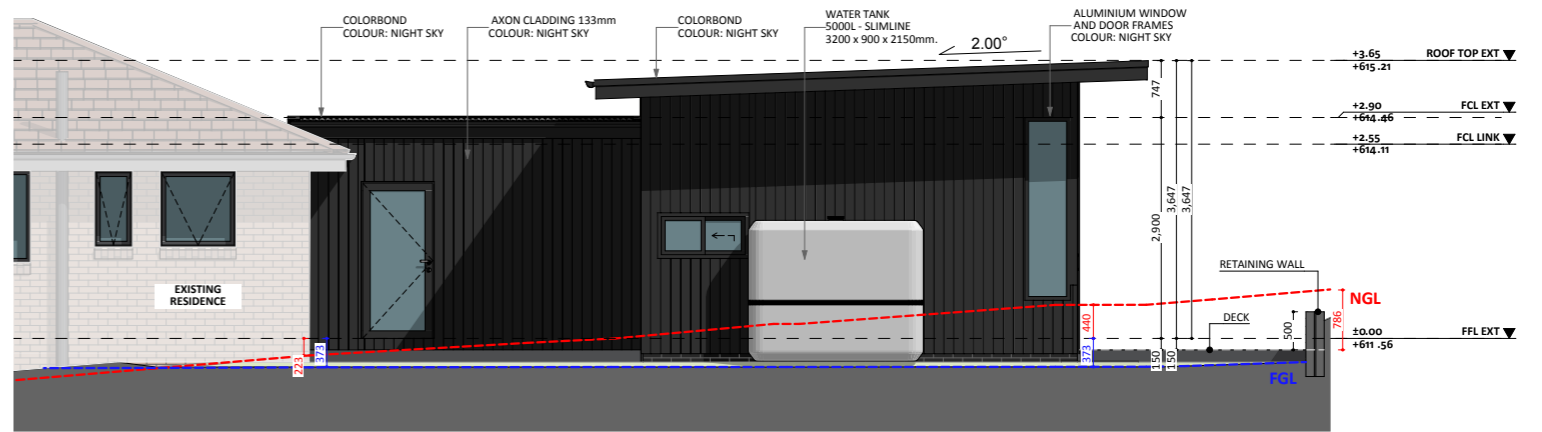
ELEVATION 04
