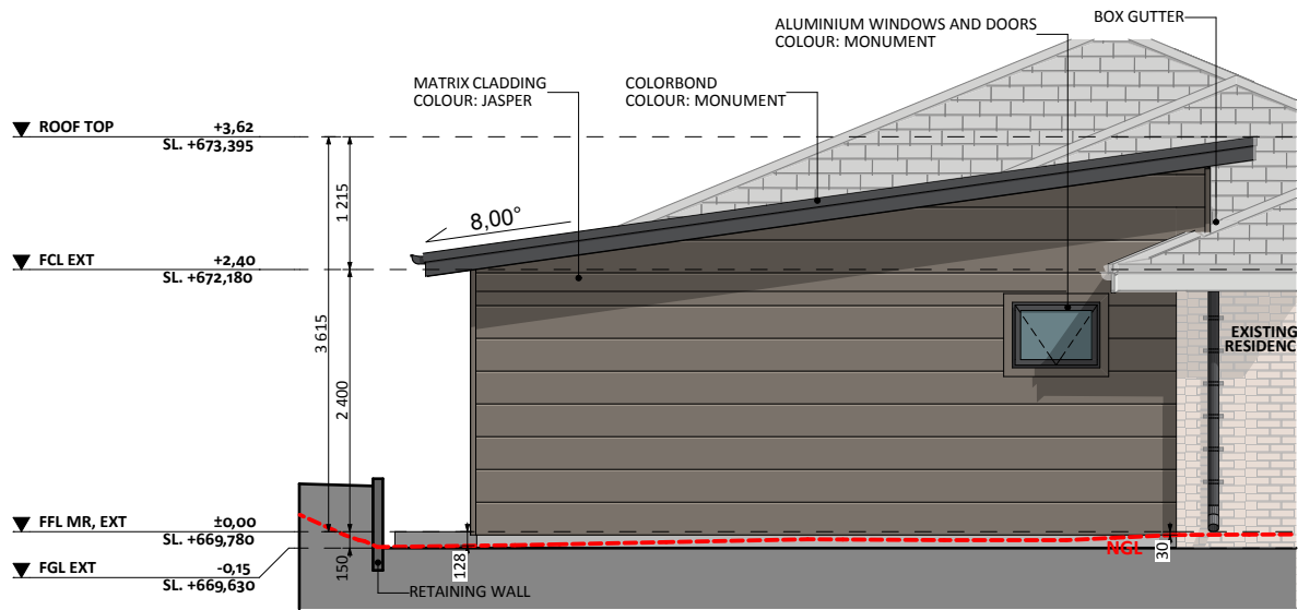
ELEVATION 01
