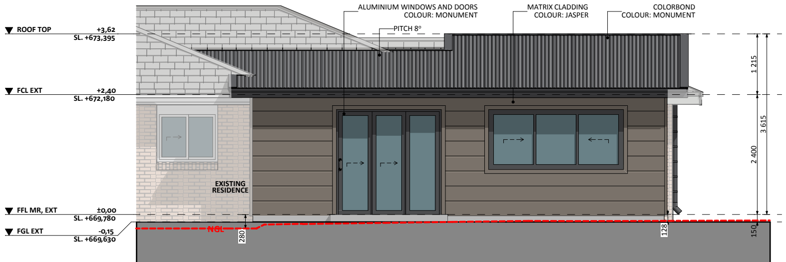
ELEVATION 02
