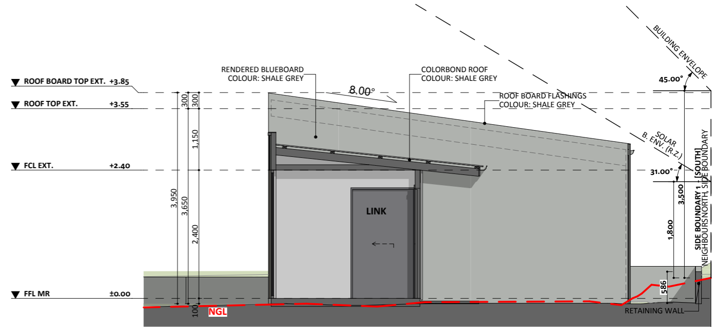
ELEVATION 2
