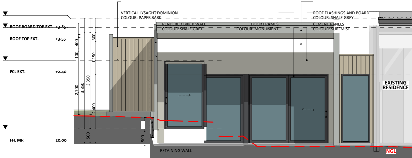
ELEVATION 1
