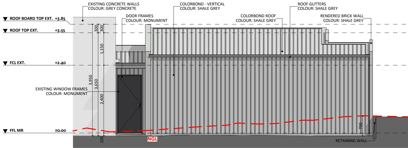
ELEVATION 3
