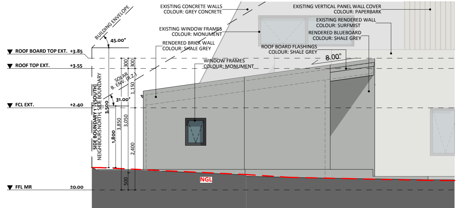
ELEVATION 4
