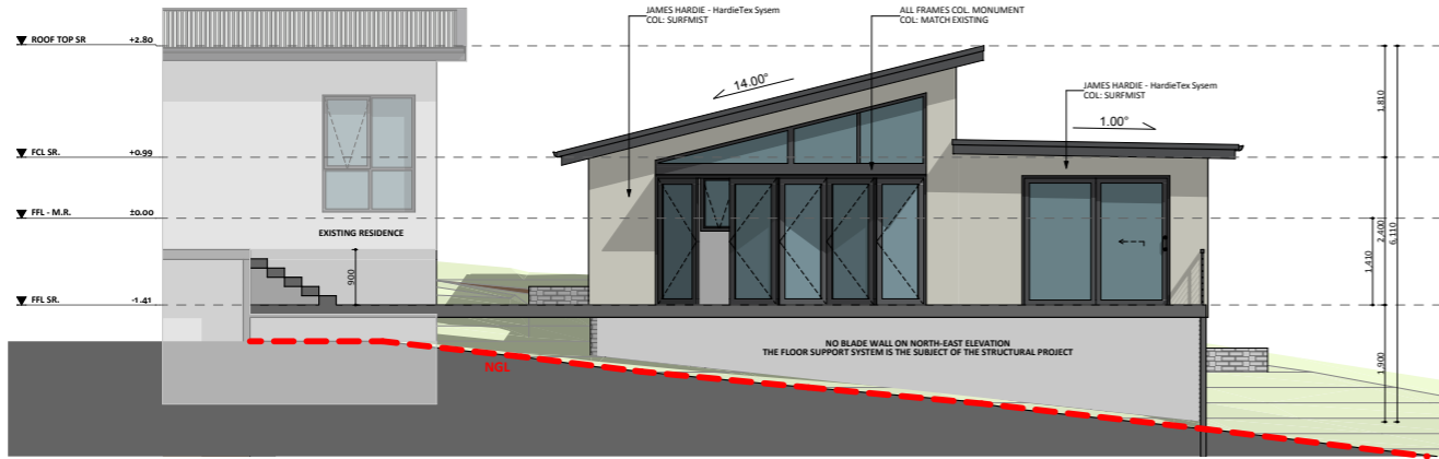
ELEVATION 01
