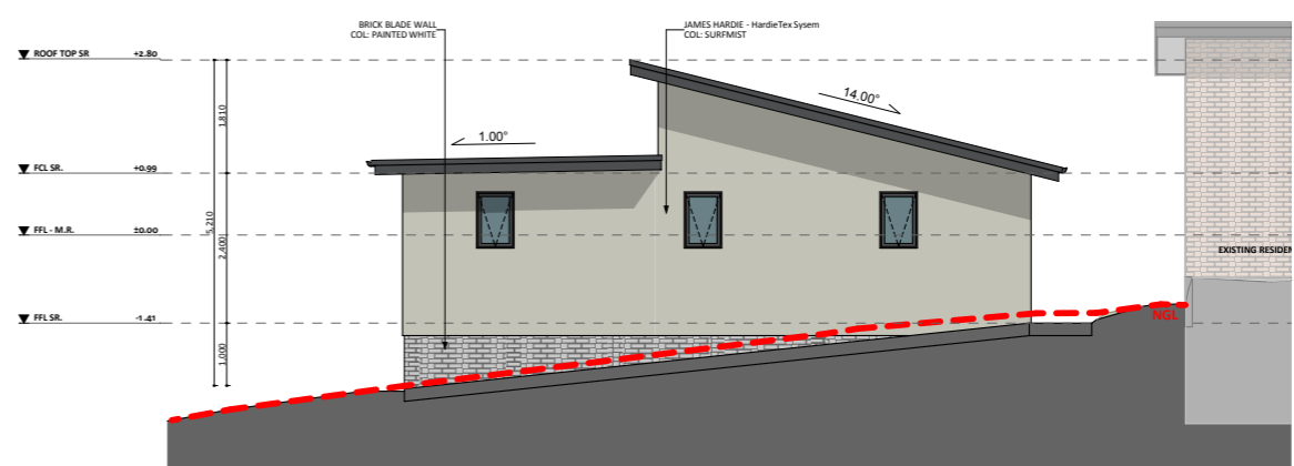
ELEVATION 02
