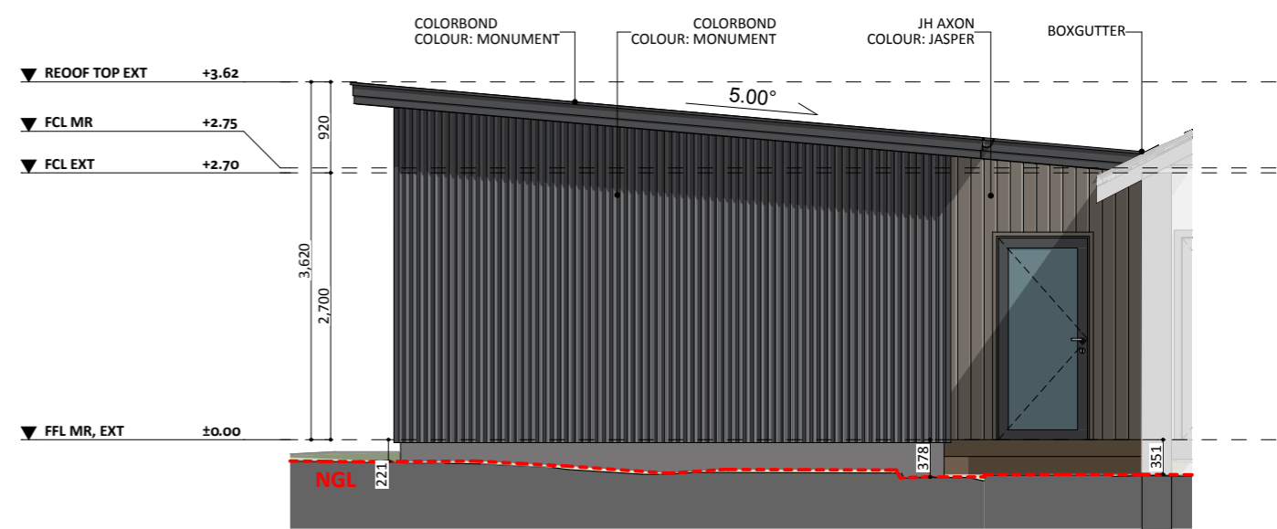
ELEVATION 04
