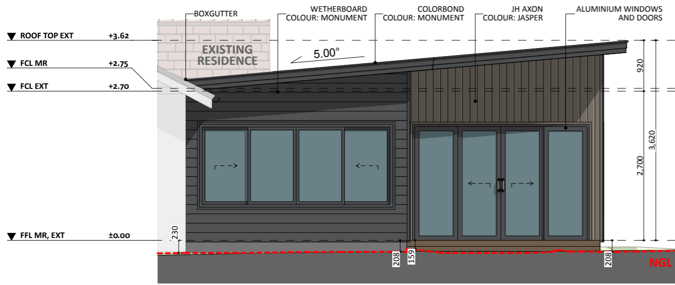
ELEVATION 01
