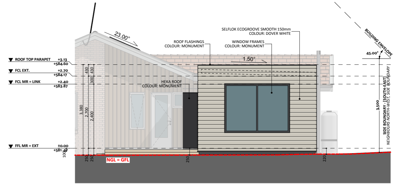
ELEVATION 02
