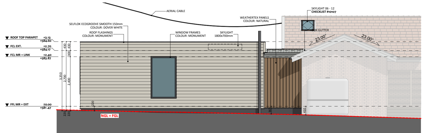
ELEVATION 04
